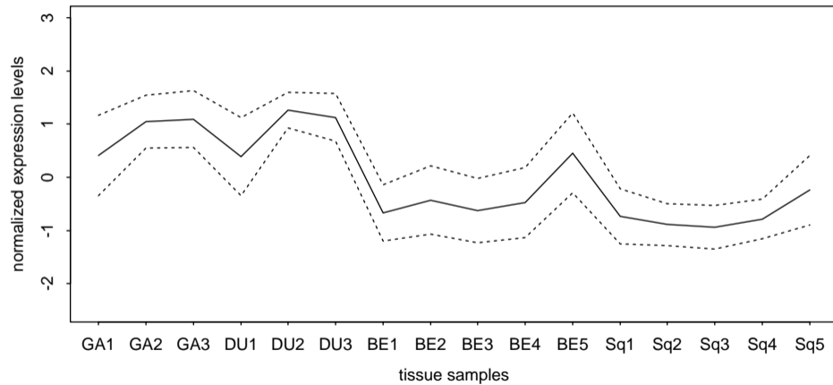
Cluster #8 (size 225)
