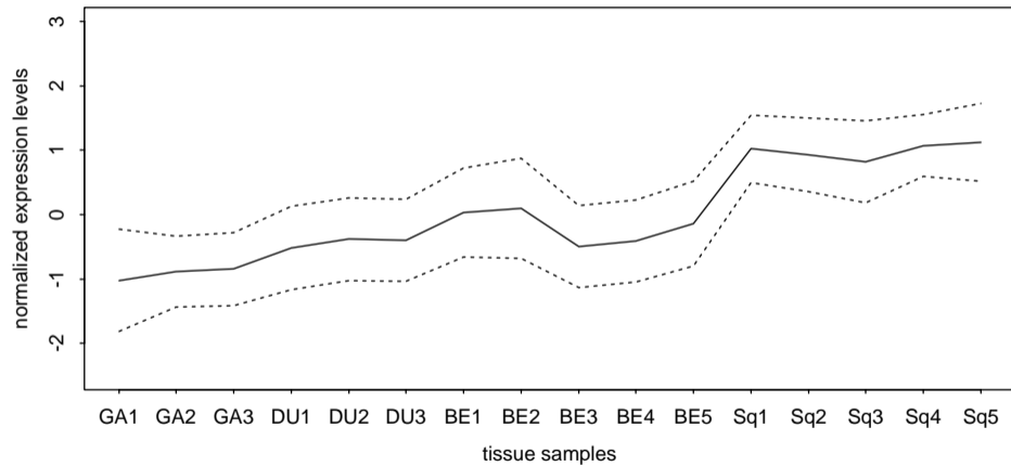
Cluster #7 (size 203)
